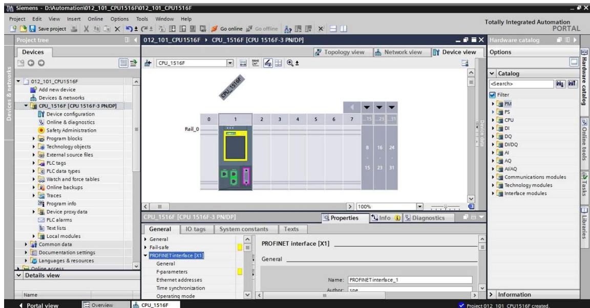
그림 3: 프로젝트 뷰
