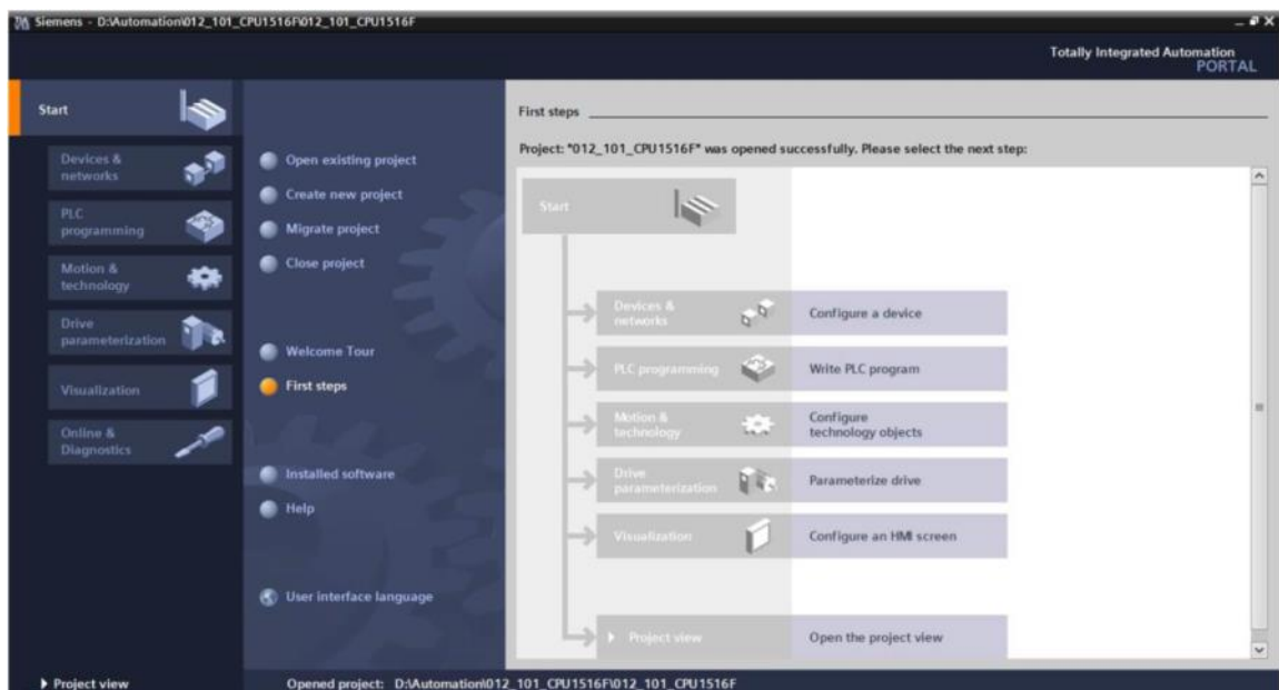
그림 2: 포털 뷰
