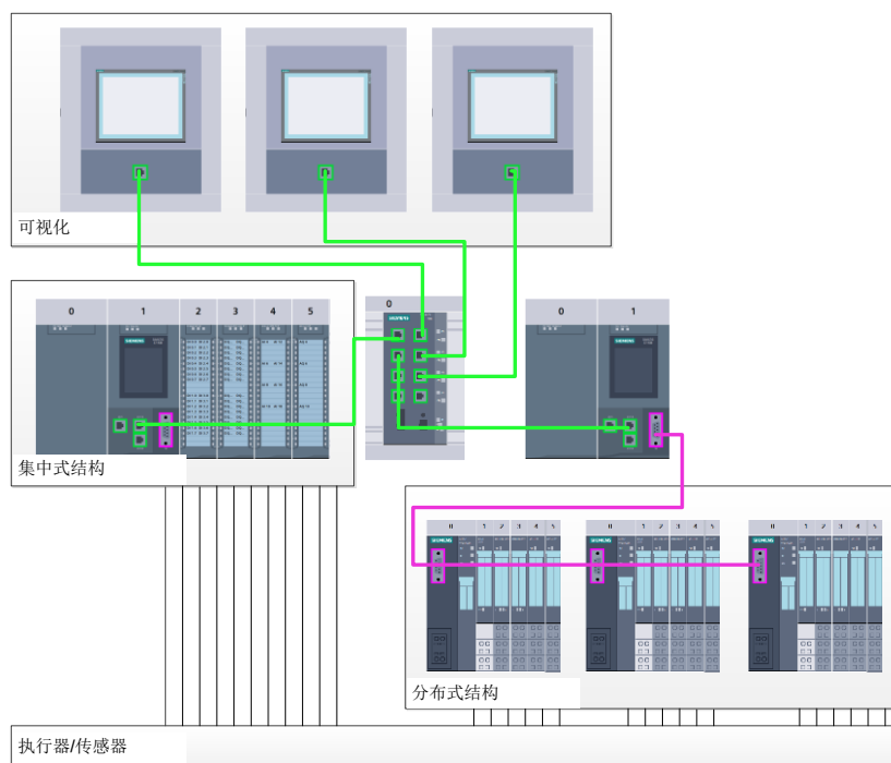
图 1: 采用集中及分散式结构的硬件配置示例
