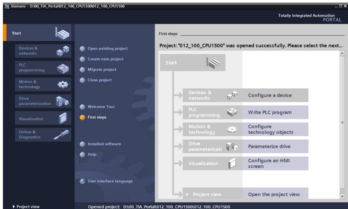
그림 2: 포털 뷰
