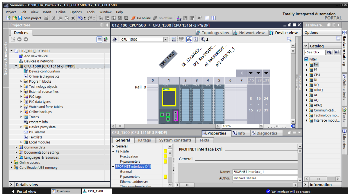
그림 3: 프로젝트 뷰
