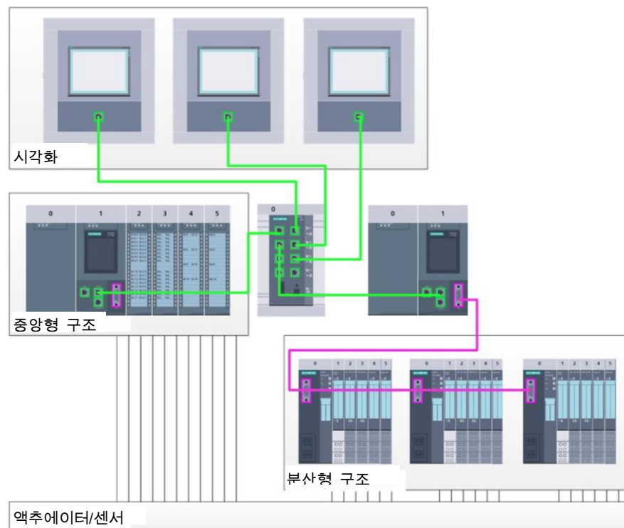
그림 1: 중앙형 및 분산형 구조를 가진 하드웨어 구성의 예
