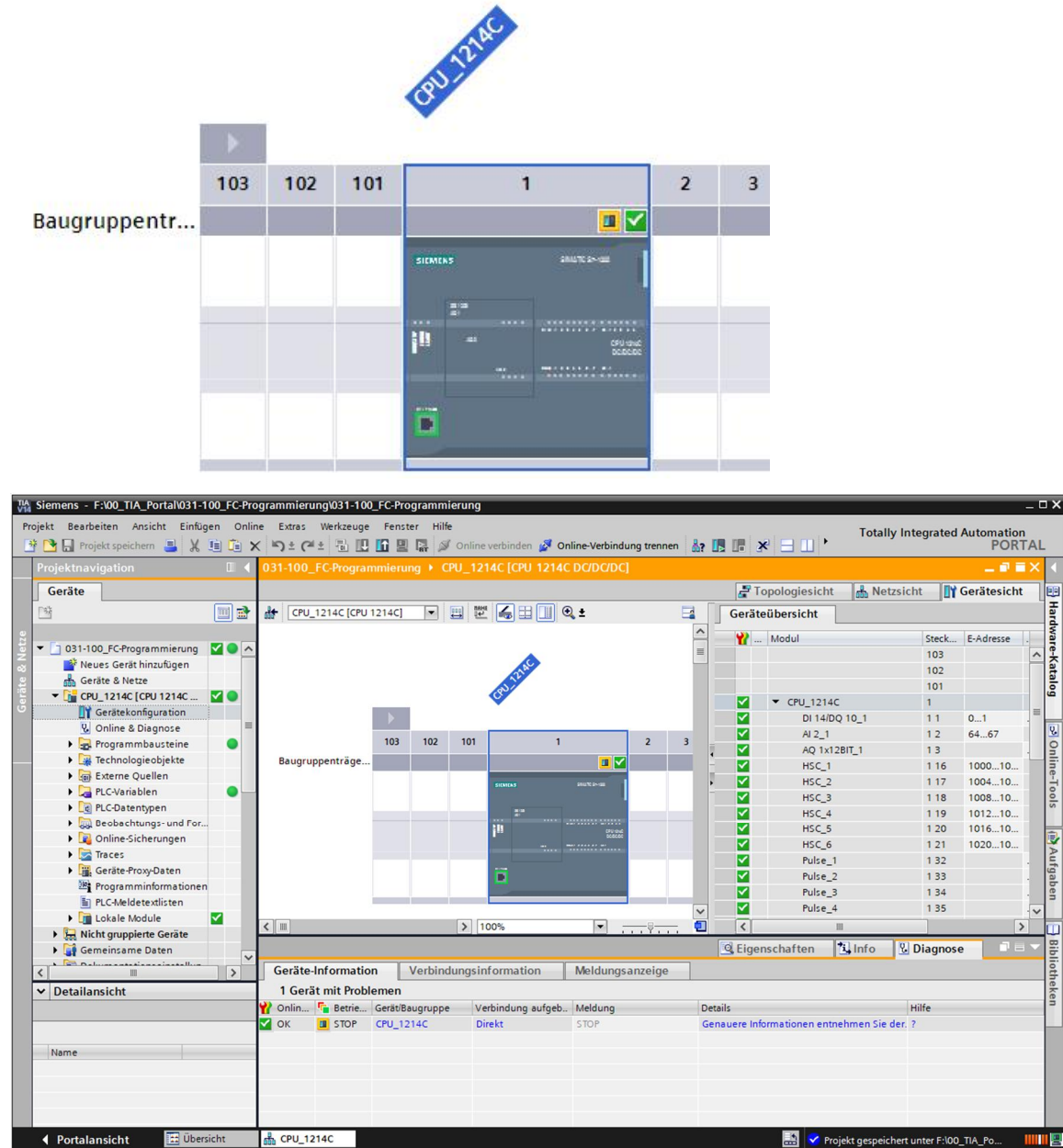
Abbildung 1: Online Ansicht der Gerätekonfiguration
