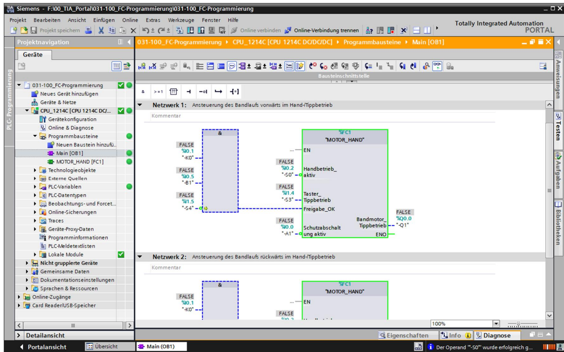
Abbildung 2: Online Ansicht des Main [OB1] Bausteins
