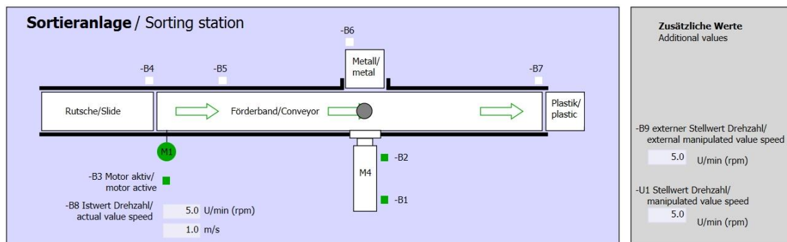
Abbildung 8: Technologieschema
