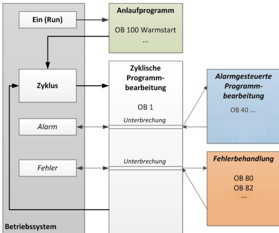
Abbildung 1: Startereignisse im Betriebssystem und OB-Aufrufe
