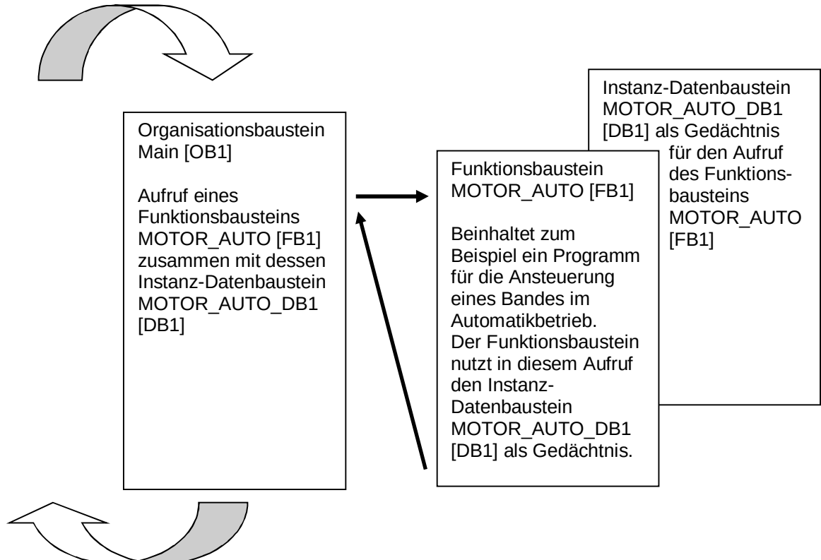
Abbildung 4: Funktionsbaustein und Instanz mit Aufruf aus dem Organisationsbaustein Main[OB1]
