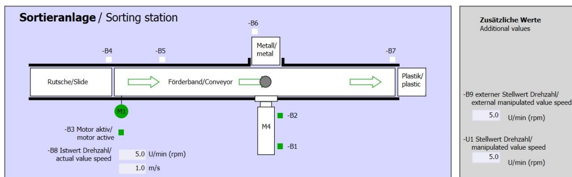
Abbildung 10: Technologieschema
