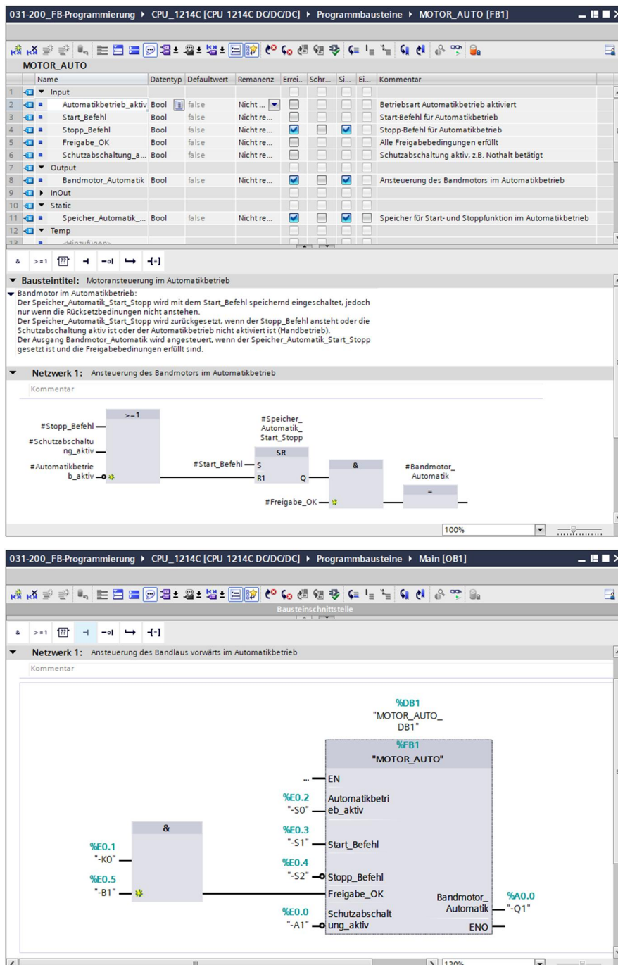
Abbildung 6: Bibliotheksfähiger Funktionsbaustein mit Aufruf im OB1
