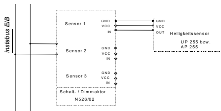
Bild 2: Montage des UP-Helligkeitssensors UP 255/01
