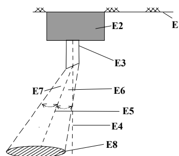
Bild 6: Erfassungskegel bei schräger Lichteintrittsfläche
