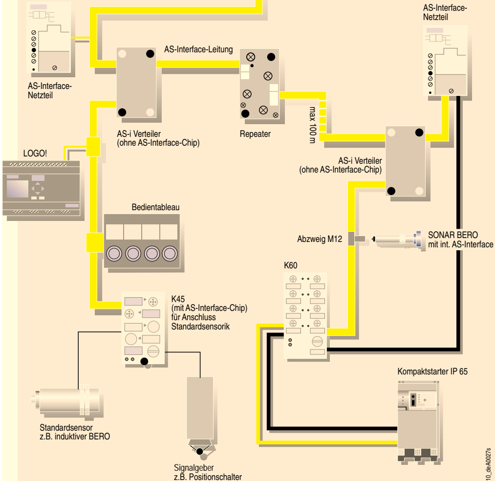
Bild 2/3 Beispiel einer Systemkonfiguration mit AS-Interface
